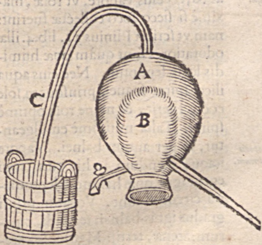
A Galea refrigeratoria, vel vesica magna qua galea vestitur, & circum isthmum arctè ligatur filo calciario.
