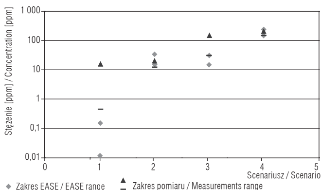
Ryc. 3. Porównanie danych pomiarowych z przewidywanymi EASE dla octanu etylu.
