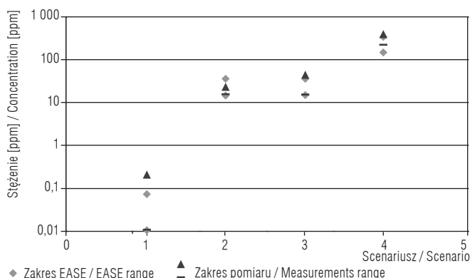
Ryc. 4. Porównanie danych pomiarowych z przewidywanymi EASE dla acetonu.
