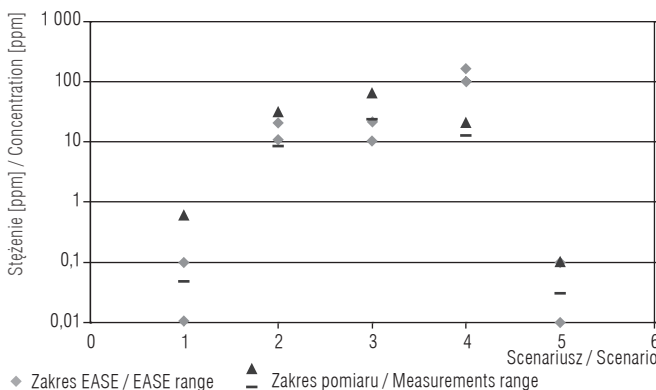
Ryc. 4. Porównanie danych pomiarowych z przewidywanymi EASE dla acetonu.
