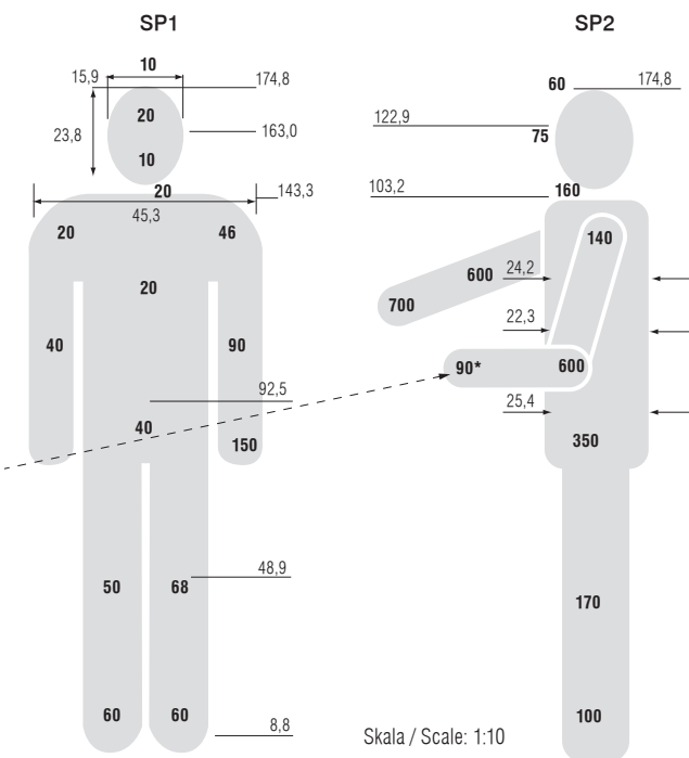
Ryc. 3. Wyniki pomiarów natężenia pola E w punktach obserwacyjnych na modelu centylowym stojącego mężczyzny o wzroście 174,8 m symulującego fizjoterapeutę podczas czynności rutynowych (SP1) i interwencyjnych (SP2) przy aparacie do diatermii KF.
