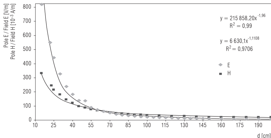
Ryc. 2. Zależność natężenia pola E i H od odległości od elektrod aparatu do diatermii KF (model Diamat G 110) — elektrody sztywne o średnicy 75 mm, nastawa 4.
