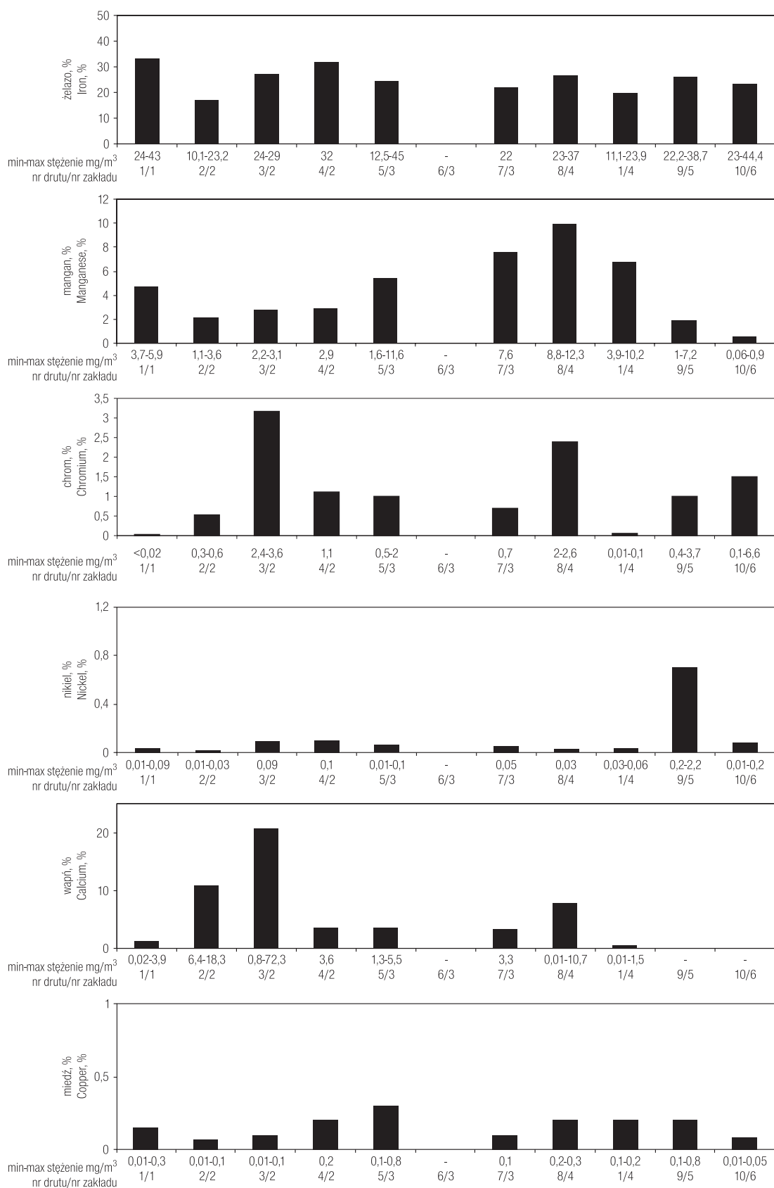
Ryc. 3. Zawartość procentowa składników w dymach na stanowiskach spawania drutami proszkowymi (objaśnienia jak w tabeli 2).
