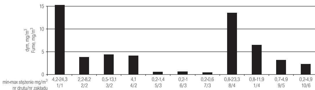
Ryc. 1. Średnie stężenia dymów na stanowiskach spawania drutami proszkowymi (objaśnienia jak w tabeli 2).
