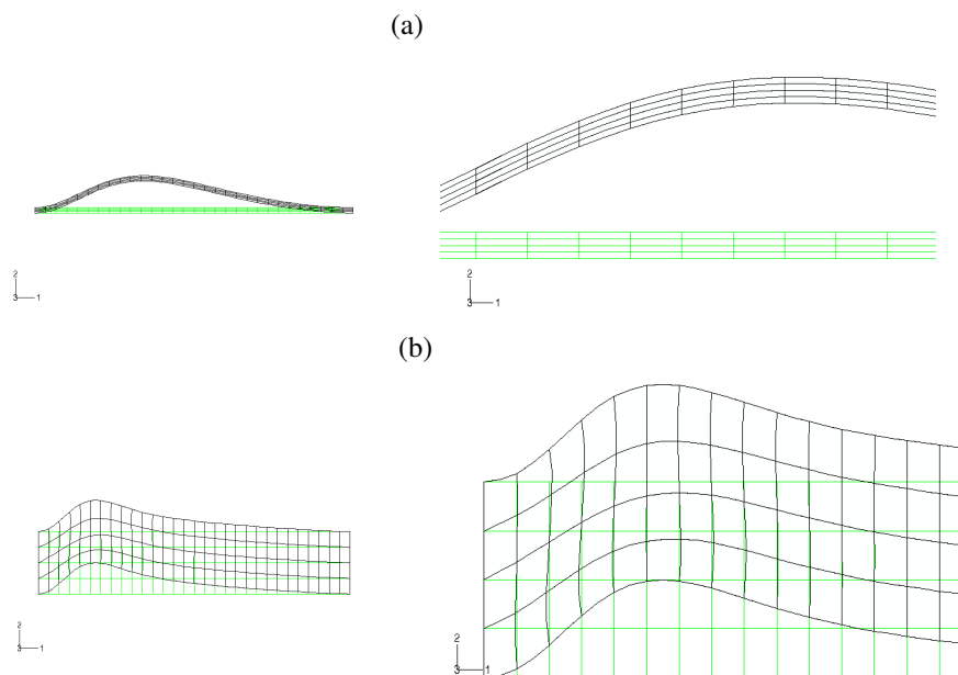
Rys. 8.9. Przemieszczenia węzłów siatek wyboczonych modeli płyt z rdzeniem ciekim (a) i grubym (b)
