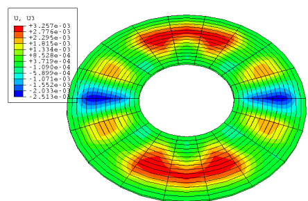
Rys. 7.17. Odpowiedź dynamiczna płyty ( G_2 = 5 MPa, h_2 = 0,01 m) z obrotowosymetrycznym m = 0 ugięciem wstępnym, ściskanej na zewnętrznym brzegu z prędkością s \approx 931 MPa/s
