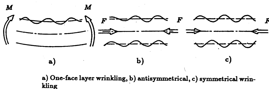
Rys. 8.6. Formy deformacji poprzecznej przedstawione w pracy [80]
