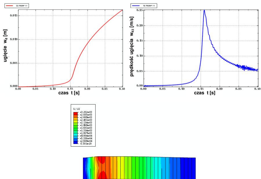
Rys. 8.13. Ugięcia i prędkości zmian ugięcia oraz postać wyboczenia płyty o parametrach: G_2 = 15,82 \text{ MPa} , h_2 = 0,06 \text{ m} , h' = 0,001 \text{ m} obciążonej na brzegu wewnętrznym
