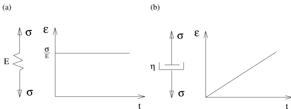
Rys. 3.5. Modele mechaniczne: (a) ciała Hooke'a, (b) cieczy Newtona
