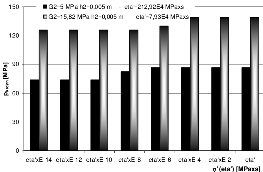
Rys. 7.14. Wpływ stałej lepkości \eta' ( \text{eta}' ) na zmiany wartości krytycznych obciążeń dynamicznych p_{krdyn} modelu MES płyty obciążonej na brzegu wewnętrznym
