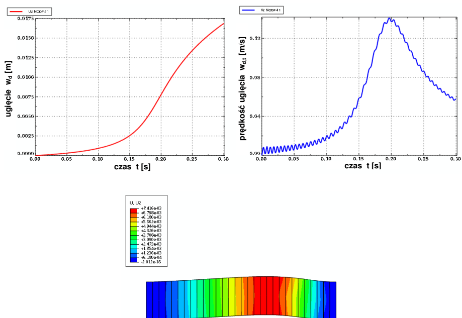
Rys. 8.12. Ugięcia i prędkości zmian ugięcia oraz postać wyboczenia płyty o parametrach: G_2 = 5 \text{ MPa} , h_2 = 0,06 \text{ m} , h' = 0,001 \text{ m} ściskanej na brzegu zewnętrznym
