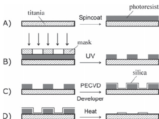
Rys. 40. Etapy tworzenia powierzchni z obszarami o różnej zwilżalności A – wytworzenie powłoki światłoczułej na ditlenku tytanu; B – naświetlanie UV przez maskę; C – wspomaganie plazmowo osadzanie z fazy gazowej \text{SiO}_2 ; D – usunięcie termiczne warstwy fotoczułej [Kanta, 2005]
