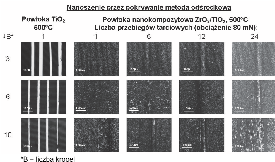
Rys. 67. Obrazy skazy po tarcii powłok ditlenku tytanu otrzymanych metodą pokrywania odśrodkowego wygrzewanych w 500°C domieszkowanych nanocząstkami \text{ZrO}_2 – wyniki z mikroskopu optycznego
