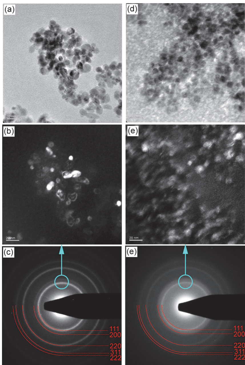
Rys. 61. Jasne (a, d) i ciemne (b, e) pola TEM nanocząstek ZrO 2 w proszku (a, b) oraz zawieszone w zolu ditlenku tytanu (d, e). Obrazom transmisyjnym odpowiadają obrazy dyfrakcyjne c i e [Piwoński, 2012]
