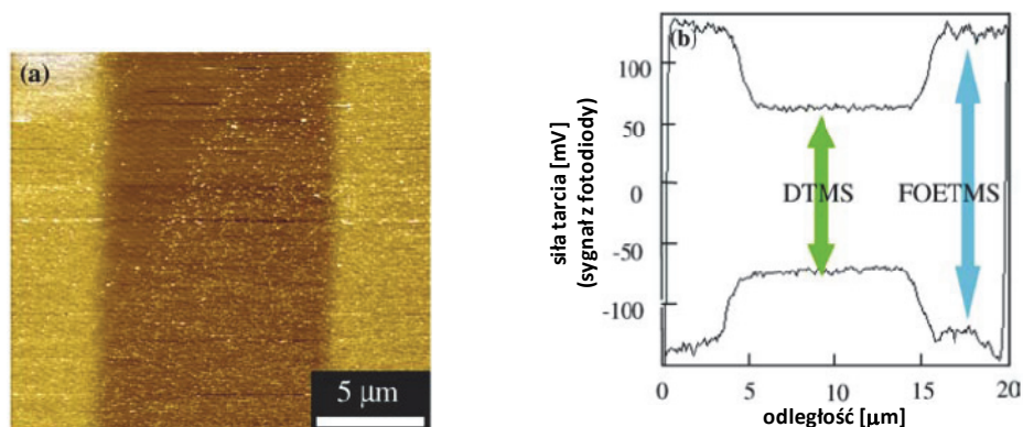
Rys. 39. Mapa sił tarcia LFM (a) oraz pętla tarcia (b) dla powierzchni krzemu zmodyfikowanej DTMS i FOETMS [Ishida, 2005]
