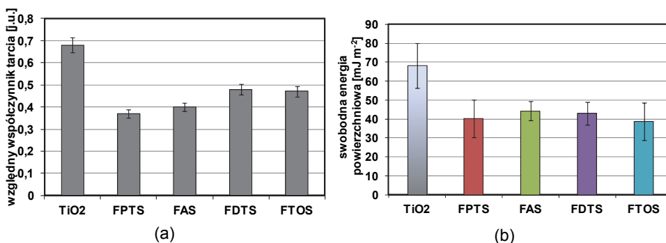
Rys. 89. Wpływ modyfikacji powierzchni na względny współczynnik tarcia (a) oraz na swobodną energię powierzchniową (b) [Piwoński 2, 2006]
