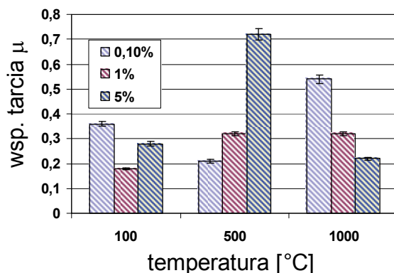
Rys. 59. Zmiany współczynnika tarcia powłok syntezowanych z 0,1%, 1% i 5% zawartością kopolimeru w wyjściowym zolu wygrzewanych w 100°C, 500°C i 1000°C
