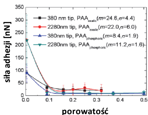
Rys. 26. Zależność sił adhezji od porowatości tlenku glinu. m – wartość siły adhezji dla poszczególnych próbek, (σ) sigma – odchylenie standartowe [Hwang, 2008]
