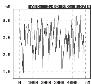
Rys. 78. Topografie powierzchni (5 \mu\text{m} \times 5 \mu\text{m} ) powłok ditlenku tytanu wygrzewanych w 100°C i zmodyfikowanych n -butylo- i n -dodecylo- ditiofosforanami cynku (ZDTP) nanoszonymi metodami LB, DC i SA [Piwoński 2, 2009]
