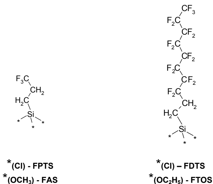
Rys. 86. Wzory strukturalne fluoroalkilosilanów: 3,3,3-trifluoropropylotrichlorosilan (FPTS), 3,3,3-trifluoropropylotrimetoksylan (FAS), 1H,1H,2H,2H-perfluorodecylo-trichlorosilan (FDTS), 1H,1H,2H,2H-perfluorodecylotrietoksylan (FTOS)
