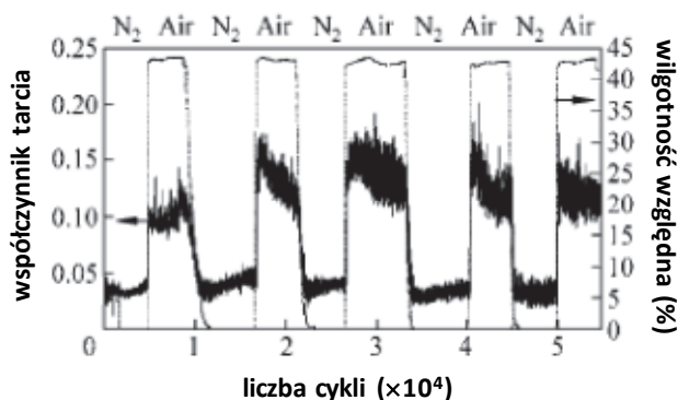
Rys. 36. Zmiany współczynnika tarcia dla powłoki typu „kameleon” YSZ/Au/MoS 2 /DLC w testach ze zmieniającą się cyklicznie wilgotnością. Odpowiedź tarciowa układu zmienia się w zależności od tego, czy składnikiem aktywnym w smarowaniu jest MoS 2 w suchym środowisku, czy też DLC w wilgotnym środowisku [Voevodin, 2005]
