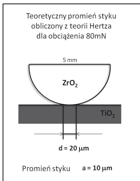
Rys. 75. Model styku tarciovego powłoki \text{TiO}_2 z przeciwpróbką – kula \text{ZrO}_2 o średnicy 5 mm
