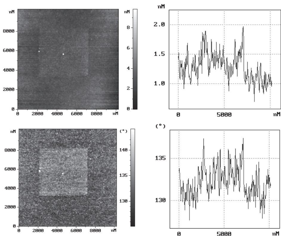
Rys. 98. Topografia powierzchni i profil oraz kontrast fazowy powłoki ditlenku tytanu wygrzewanej w temperaturze 500°C
