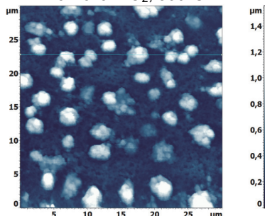
Powłoka nanokompozytowa \text{TiO}_2 + \text{ZrO}_2 , 500°C
