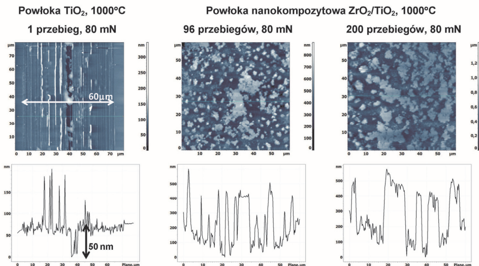
Rys. 73. Obrazy AFM skaz po tarcu powłok ditlenku tytanu wytwarzanych metodą nakładania przez pokrywanie odśrodkowe wygrzewanych w 1000°C bez nanocząstek oraz domieszkowanych nanocząstkami (deponowanych z trzech kropli) [Piwoński, 2012]
