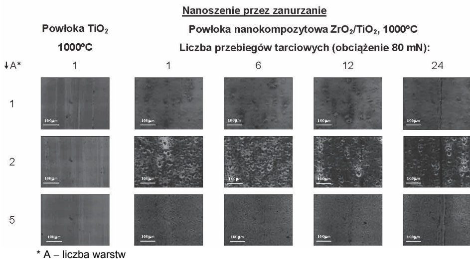
Rys. 70. Obrazy skaz po tarcii powłok ditlenku tytanu domieszkowanych nanocząstkami ditlenku cyrkonu, otrzymanych przez zanurzanie po wygrzaniu w 1000°C – wyniki z mikroskopu optycznego
