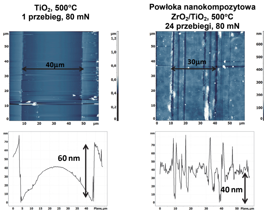
Rys. 66. Obrazy AFM skaz po tarcii powłoki \text{TiO}_2 500°C oraz powłoki \text{TiO}_2 500°C z nanocząstkami \text{ZrO}_2 naniesionych metodą przez zanurzenie
