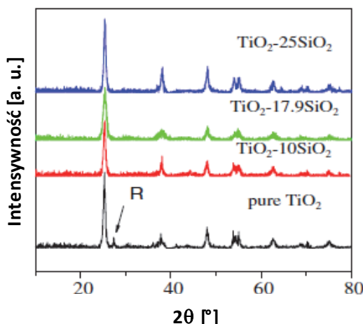
Rys. 16. Dyfraktogramy powłok \text{TiO}_2 z różną zawartością \text{SiO}_2 wygrzewane w temp. 500^\circ\text{C} przez 4 h [Jia, 2007]
