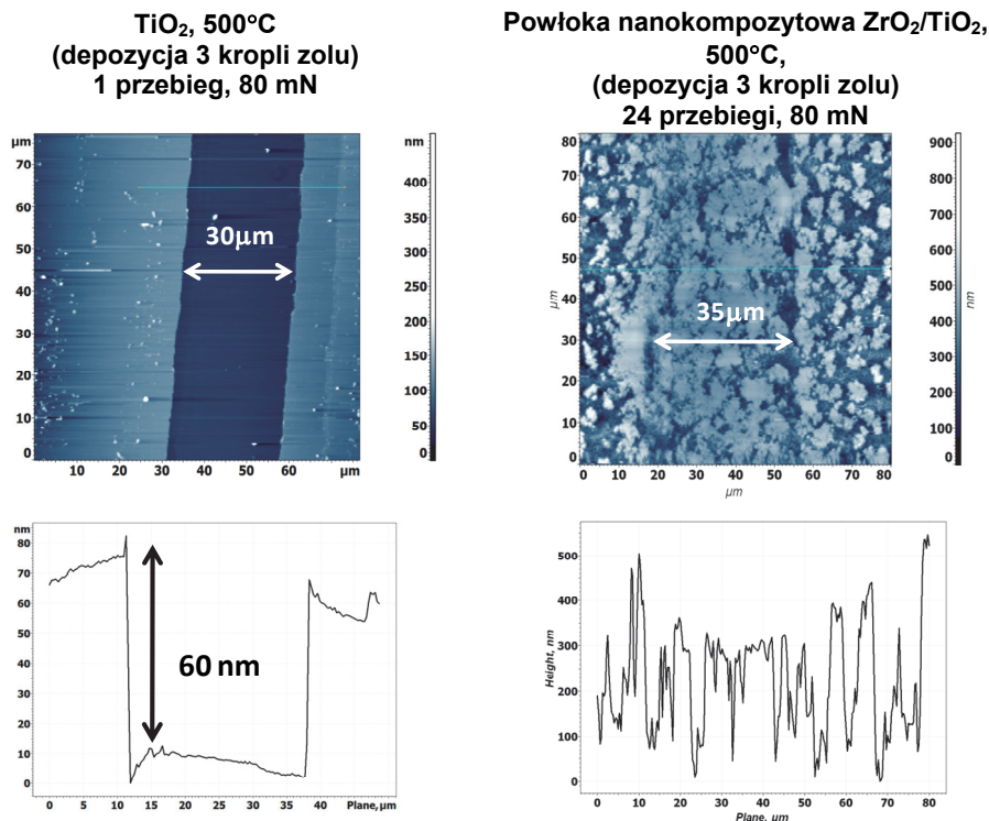
Rys. 68. Obrazy AFM skaz po tarcii na powłoce ditlenku tytanu oraz na powłoce kompozytowej ditlenku tytanu z nanocząstkami ditlenku cyrkonu. Obie powłoki naniesiono metodą pokrywania odśrodkowego i wygrzano w 500°C
