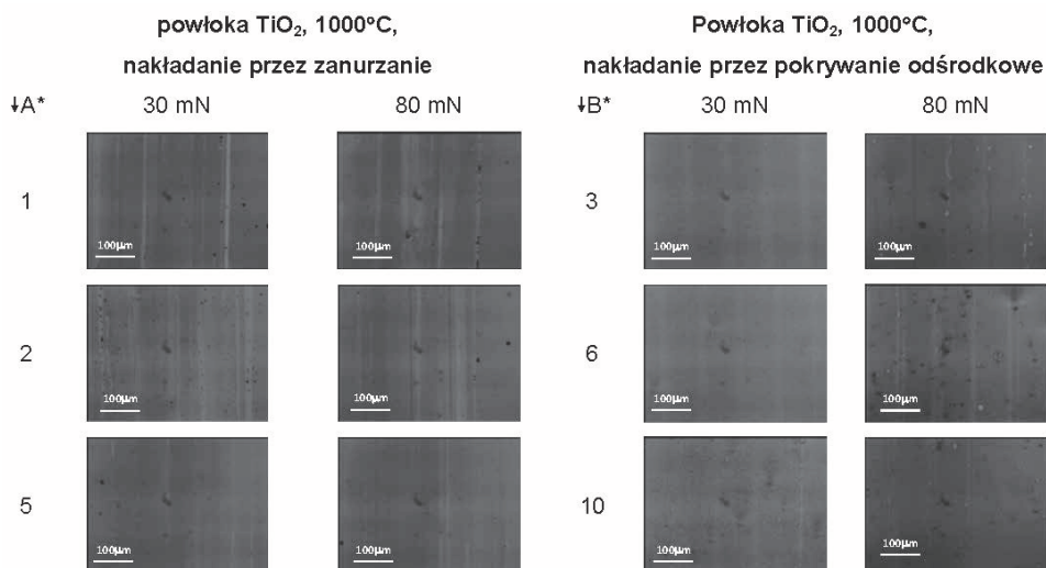
Rys. 69. Porównanie wytrzymałości na zużycie powłok ditlenku tytanu bez nanocząstek wygrzewanych w 1000°C w zależności od liczby naniesionych warstw (nakładanie przez zanurzanie), liczby zdeponowanych kropli (nakładanie przez pokrywanie odśrodkowe) oraz obciążenia – zdjęcia z mikroskopu optycznego
