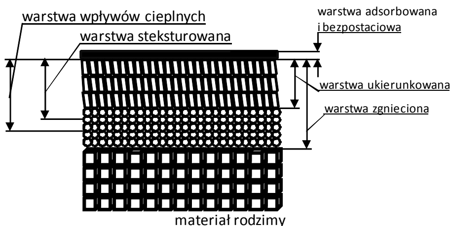
Rys. 1. Model powłoki wg Hebda i Wachala [Hebda, 1980]
