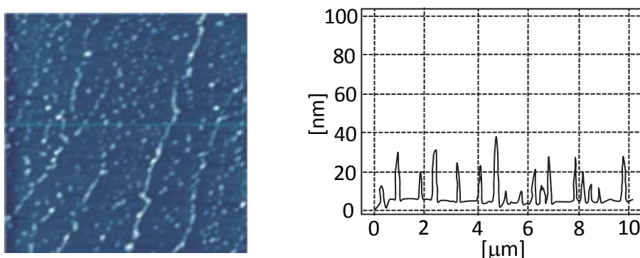
Rys. 60. Obraz AFM (10 μm x 10 μm) nanocząstek \text{ZrO}_2 zdeponowanych na powierzchni krzemu wraz z profilem przekroju
