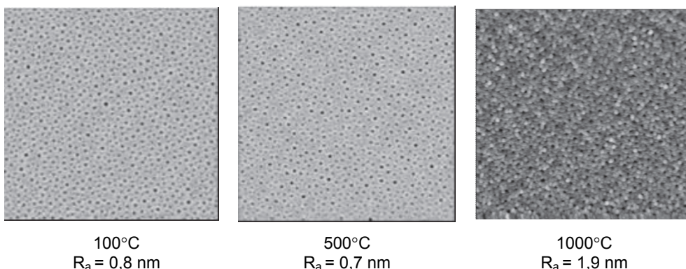
Rys. 58. Obrazy AFM ( 5,5\mu\text{m} \times 5,5\mu\text{m} ) powłoki ditlenku tytanu przygotowanej z kopolimerem blokowym o stężeniu 0,1% w zolu, po wygrzewaniu w 100°C, 500°C i 1000°C
