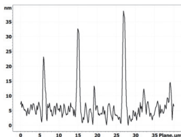
Rys. 74. Porównanie topografii powierzchni powłok ditlenku tytanu oraz powłok ditlenku tytanu zawierających nanocząstki otrzymanych metodą nanoszenia przez zanurzenie lub metodą nakładania przez pokrywanie odśrodkowe [Piwoński, 2012]
