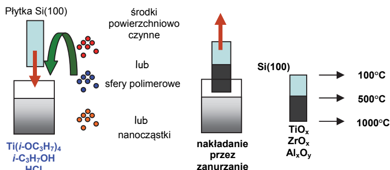
Rys. 45. Ogólny schemat wytwarzania powłok ceramicznych zol-żel tlenków tytanu i innych tlenków metodą przez zanurzanie na płytkach krzemowych
