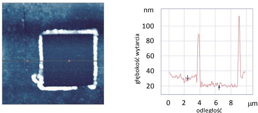
Rys. 81. Obraz AFM (10 μm x 10 μm) oraz profil przekroju śladu wytarcia powstałego w wyniku skanowania ostrzem AFM powierzchni ditlenku tytanu zmodyfikowanego kwasem HDTP C 16 metodą DC
