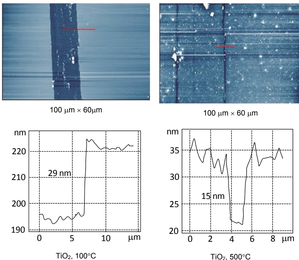
Rys. 53. Obrazy AFM skaz powstałych po tarcia oraz profile ich przekroju dla powłok \text{TiO}_2 wygrzewanych w 100°C i 500°C
