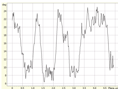
Rys. 95. Topografia i kontrast fazowy powłok ditlenku tytanu po modyfikacji tlenkiem etylenem w fazie gazowej
