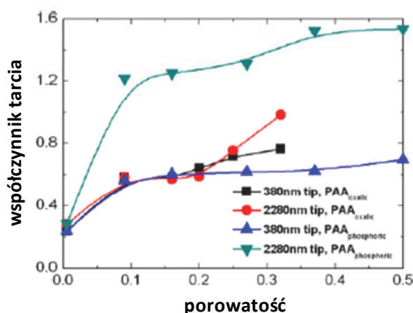
Rys. 28. Zależność wsp. tarcia od porowatości dla różnych promieni sond skanujących [Hwang, 2008]
