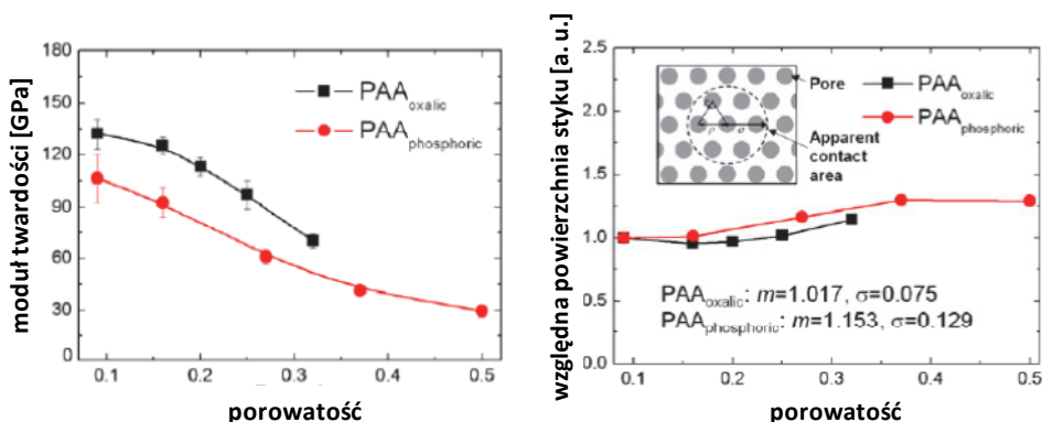
Rys. 27. Moduł twardości – (rys. lewy) oraz względna powierzchnia styku (rys. prawy) przybliżona przez teorie Hertza i wgłębiania w funkcji porowatości [Hwang, 2008] PAA oxalic or PAA phosphoric – porous anodic alumina – tlenek glinu wytwarzany na drodze utleniania anodowego w obecności kwasów szczawiowego lub fosforowego
