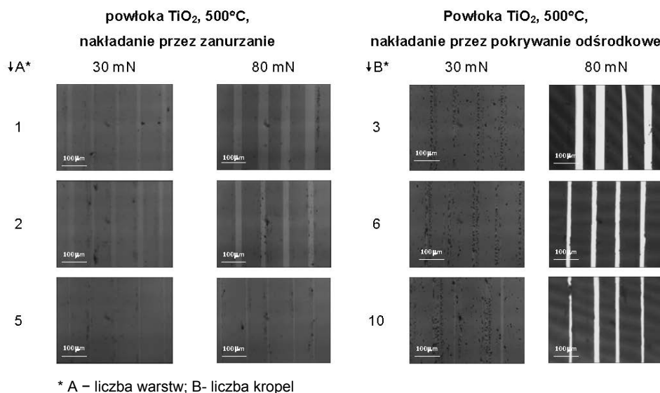
Rys. 64. Porównanie wytrzymałości na zużycie powłok ditlenku tytanu bez nanocząstek wygrzewanych w 500°C w zależności od liczby naniesionych warstw (nanoszenie przez zanurzenie), liczby zdeponowanych kropli (nakładanie przez pokrywanie odśrodkowe) oraz obciążenia – zdjęcia z mikroskopu optycznego
