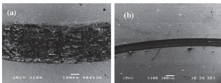
Rys. 12. Obrazy SEM śladów zużycia powstałych na powierzchni powłoki Ti (a) oraz utlenionej powłoki Ti (b) przy obciążeniu 1 N [Krishna, 2005]
