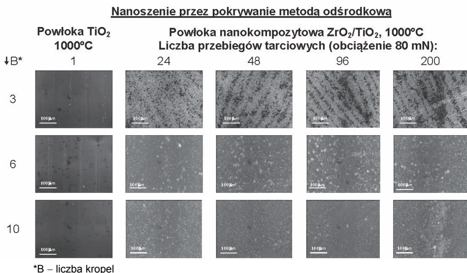
Rys. 72. Obrazy skaz po tarcii powłok ditlenku tytanu otrzymanych metodą nakładania przez pokrywanie odśrodkowe wygrzewanych w 1000°C domieszkowanych nanocząstkami – wyniki z mikroskopu optycznego [Piwoński, 2012]
