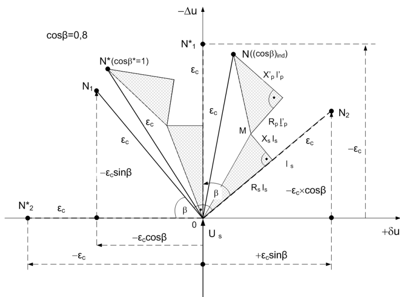
Rys. 5.8. Diagram Möllingera-Gewecke ilustrujący graniczne położenia odcinka odpowiadającego procentowej wartości błędu całkowitego \varepsilon_c (patrz rys. 5.3)
