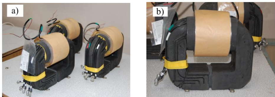
Rys. 4.3. Niskonapięciowe modele przekładnika napięciowego SN (Przekładnik fabryczny: U_{pn} = 22/\sqrt{3} \text{ kV} ; U_{sn} = 110/\sqrt{3} \text{ V} i 110/3 \text{ V} )
