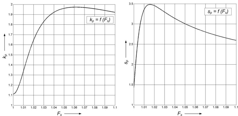
Rys. 5.12. Współczynnik kształtu k_p i szczytu s_p prądu pierwotnego w funkcji współczynnika F_s ( c_L = 256 ) (przebiegi otrzymane metodą analityczną)
