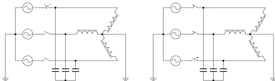
Rys. 6.11. Przykładowe układy SN sprzyjające oscylacjom ferorezonansowym [57] (zaznaczono pojemności systemu i uzwojenia G_N transformatora SN/nn)
