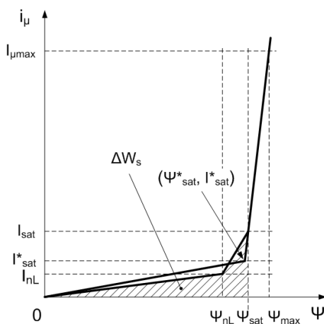
Rys. 6.15. Charakterystyka magnesowania rdzenia ferromagnetycznego przekładnika (aproksymacja trójodcinkowa i równoważna energetycznie aproksymacja dwuodcinkowa)
