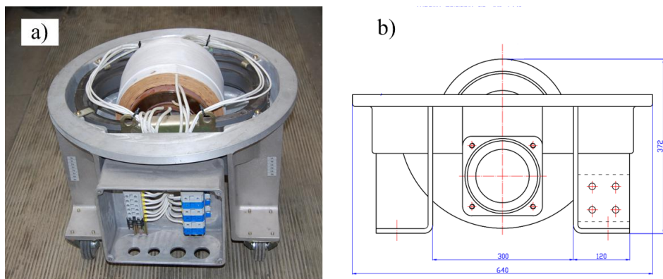
Rys. 4.1. Niskonapięciowy model równoważny przekładnika napięciowego WN (Przekładnik fabryczny: U_{pn} = 110/\sqrt{3} \text{ kV} ; U_{sn} = 100/\sqrt{3} \text{ V} i 100/3 \text{ V} ): a) zdjęcie konstrukcji modelu, b) podstawowe wymiary zewnętrzne
