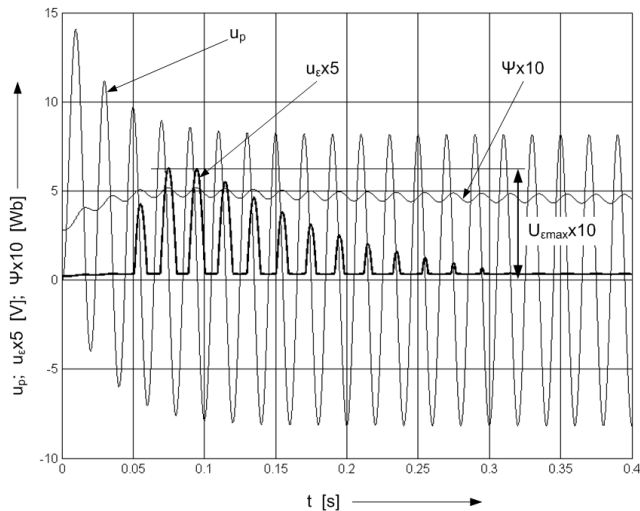
Rys. 5.25. Przebiegi napięcia pierwotnego, strumienia skojarzonego z obwodem wtórnym i napięcia błędu otrzymane metodą symulacji komputerowej dla równoważnego niskonapięciowego modelu przekładnika WN (rozdz. 4.1.1) ( T_p = 30 ms; T_\mu = 16 s; \Psi_s = 0,485 Wb; i_\mu(0) = I_{\mu max} )
