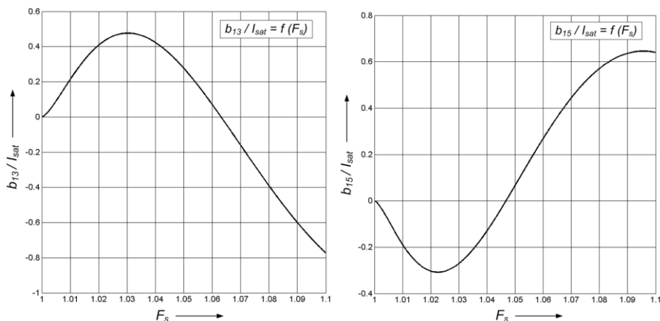
Rys. 5.18. Współczynniki b_{13} i b_{15} rozwinięcia w szereg Fouriera funkcji opisującej przebieg prądu pierwotnego dla przepięcia ustalonego wywołującego słaby stan nasycenia obwodu magnetycznego, odniesione do prądu granicznego nasycenia I_{sat} , w funkcji współczynnika F_s ( c_L = 256 ) (przebiegi otrzymane metodą analityczną)
