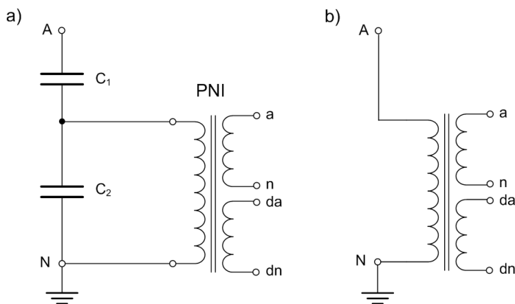
Rys. 1.1. Układy dwóch podstawowych typów jednofazowych przekładników napięciowych WN: a) przekładnik pojemnościowy, b) przekładniki indukcyjny
