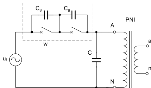
Rys. 6.9. Schemat układu jednej fazy wyłącznika ( w ) z pojemnościami sterującymi ( C_g ) włączonymi szeregowo z przekładnikiem napięciowym indukcyjnym ( PNI ) C – pojemność wypadkowa jednej fazy między systemem szyn a ziemią
