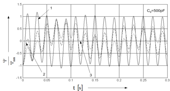
Rys. 6.17. Względna wartość chwilowa strumienia skojarzonego (odniesiona do amplitudy strumienia przy napięciu U_p = U_{pn} ); \varphi_u = 0 ; C_g = 500 \text{ pF} ( 1 \rightarrow c = 0 ; 2 \rightarrow c = 1 ; 3 \rightarrow c = 2 )
