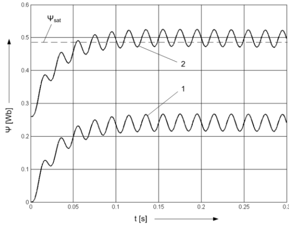
Rys. 5.24. Przebieg strumienia skojarzonego z obwodem wtórnym równoważnego modelu niskonapięciowego przekładnika WN:
