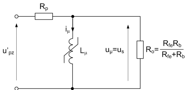
Rys. 5.23. Schemat zastępczy przekładnika do analizy pracy w stanie przejściowym (wszystkie wielkości sprowadzono do strony wtórnej) R_o – wypadkowa rezystancji obciążenia R_b i rezystancji R_{fe} odwzorowującej strat mocy czynnej w rdzeniu ferromagnetycznym; R_s \approx 0 ( R_s \ll R_o )
