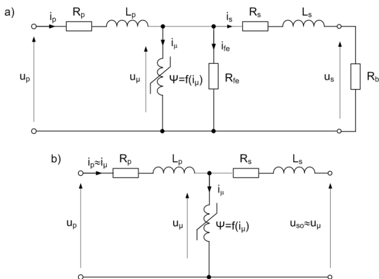
Rys. 5.9. Pełny (a) i uproszczony dla stanu przebiecia ustalonego (b) schemat zastępczy przekładnika napięciowego indukcyjnego (wszystkie wielkości sprowadzono do strony pierwotnej)
