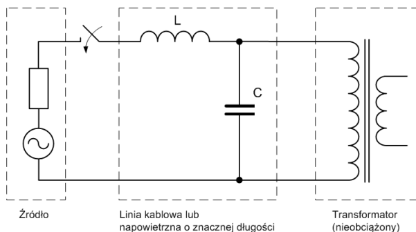
Rys. 6.12. Schematyczna ilustracja układu jednej fazy nieobciążonego transformatora mocy zasilanego za pośrednictwem linii o znacznej pojemności (C) ( L – skupiony parametr odwzorowujący indukcyjność linii)
