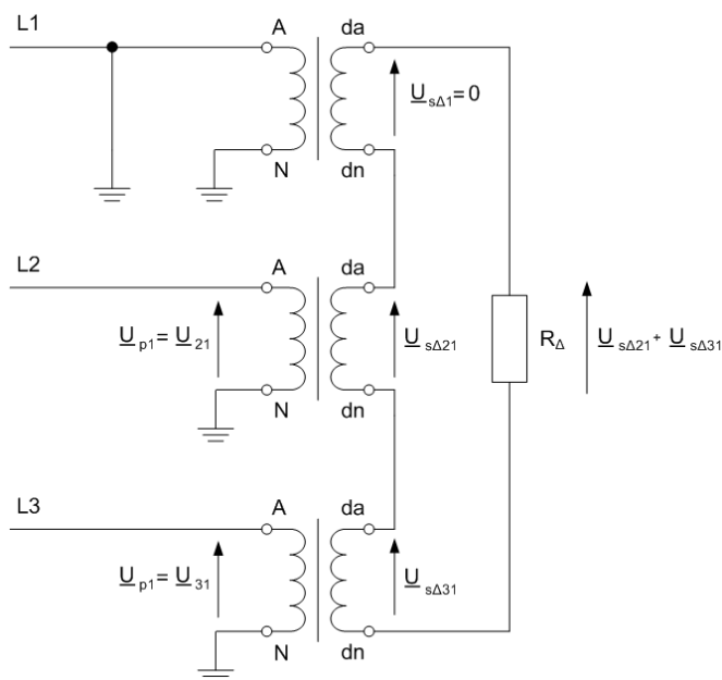
Rys. 7.4. Przekładniki napięciowe indukcyjne z uzwojeniami dodatkowymi obciążonymi rezystorem R_{\Delta} w sieci SN przy zwarcu doziemnym jednej fazy
