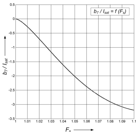
Rys. 5.16. Współczynniki b_5 i b_7 rozwinięcia w szereg Fouriera funkcji opisującej przebieg prądu pierwotnego dla napięcia ustalonego wywołującego słabe nasycenie obwodu magnetycznego, odniesione do prądu granicznego nasycenia I_{sat} , w funkcji współczynnika F_s ( c_L=256 ) (przebiegi otrzymane metodą analityczną)
