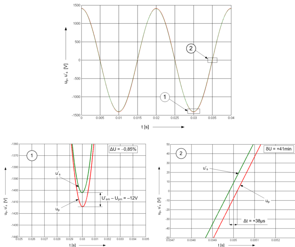
Rys. 5.7. Przebiegi czasowe napięć otrzymane metodą symulacji komputerowej w trybie zwykłym oraz w trybach: „Zoom1” i „Zoom2”
