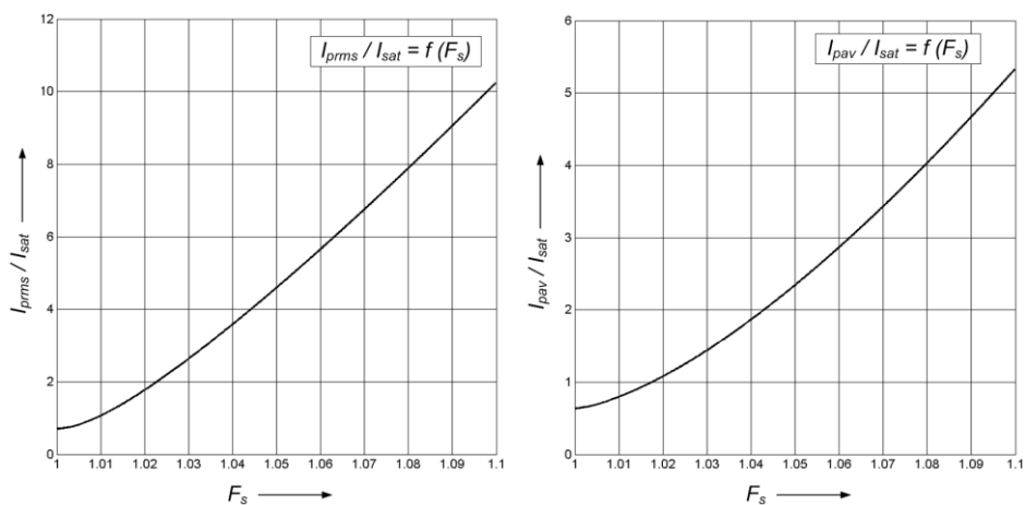
Rys. 5.11. Odniesiona do prądu granicznego nasycenia I_{sat} wartość skuteczna I_{prms} i średnia z modułu I_{pav} prądu pierwotnego w funkcji współczynnika F_s ( c_L = 256 ) (przebiegi otrzymane metodą analityczną)
