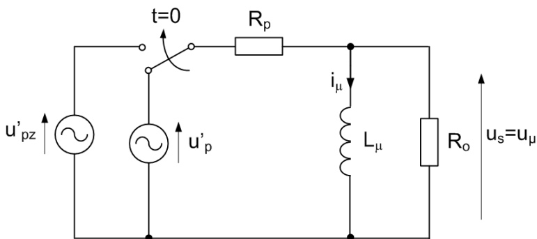
Rys. D1. Schemat układu do obliczenia prądu magnesującego (strumienia skojarzonego) w stanie przejściowym przy zwarcie w systemie (wszystkie wielkości sprowadzono do strony wtórnej)
