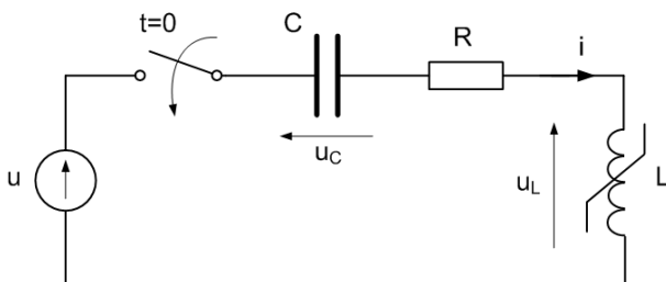
Rys. 6.4. Schemat podstawowego układu szeregowego z nieliniowym elementem indukcyjnym L pobudzonego w chwili t = 0 do oscylacji ferorezonansowych w wyniku dołączenia napięciowego źródła energii elektrycznej
