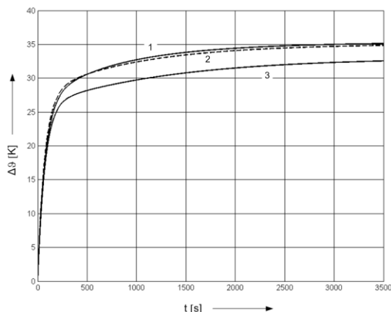
Rys. 5.43. Przebiegi przyrostów temperatury \Delta\theta dla pracy ciągłej (1 – uzwojenie pierwotne, 2 – uzwojenie wtórne, 3 – rdzeń)
