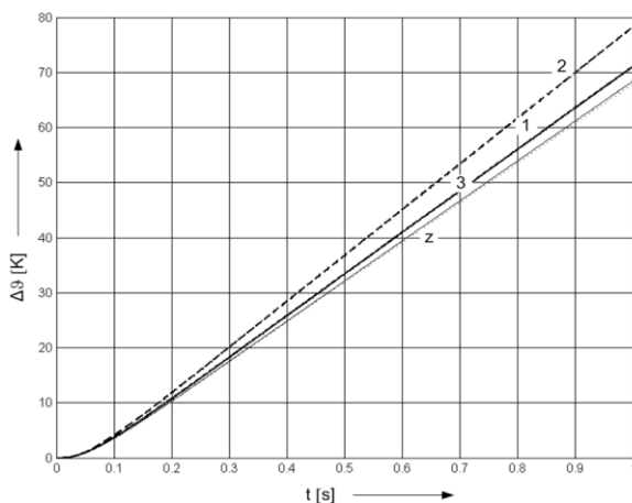
Rys. 5.44. Przebiegi przyrostów temperatury \Delta\theta dla pracy krótkotrwałej (1,2,3 – jak na rys. 5.43; z – powierzchnia zewnętrzna izolacji żywicznej)
