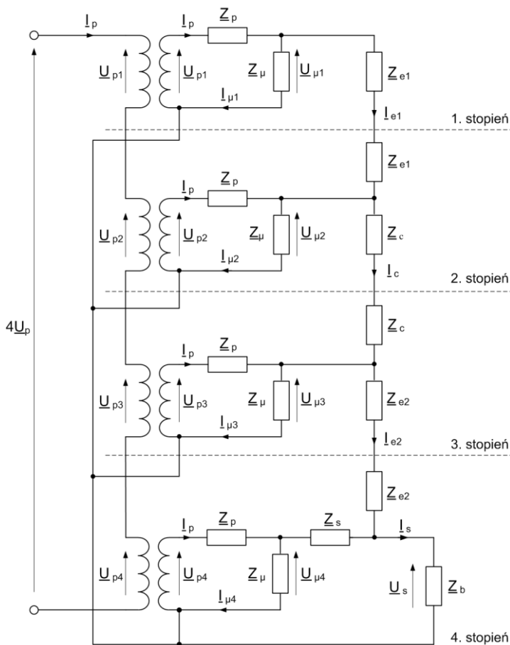
Rys. 5.3. Schemat zastępczy kaskadowego przekładnika napięciowego indukcyjnego o czterostopniowym, dwurdzeniowym rozwiązaniu konstrukcyjnym (wszystkie wielkości sprowadzono do strony wtórnej)
