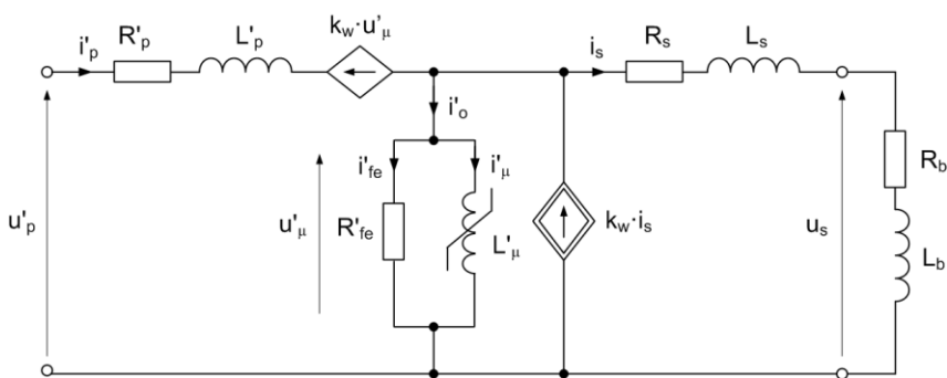
Rys. 5.1. Schemat zastępczy przekładnika napięciowego indukcyjnego z uwzględnieniem korekcji zwojowej (wszystkie wielkości sprowadzono do strony wtórnej)
