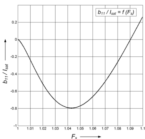
Rys. 5.17. Współczynniki b_9 i b_{11} rozwinięcia w szereg Fouriera funkcji opisującej przebieg prądu pierwotnego dla napięcia ustalonego wywołującego słabe nasycenie obwodu magnetycznego, odniesione do prądu granicznego nasycenia I_{sat} , w funkcji współczynnika F_s ( c_L=256 ) (przebiegi otrzymane metodą analityczną)
