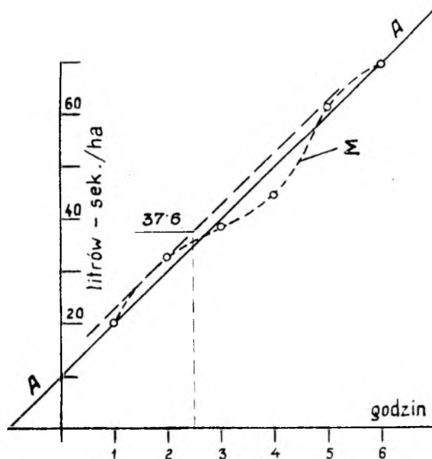
Rys. 3. Sumowane średnie natężenie w dorzeczu wyrównane prostą A-A
