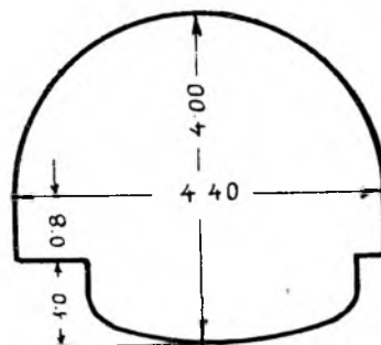
Rys. 5). Potrzebny przekrój końcowy kolektora lewobrzeżnego
