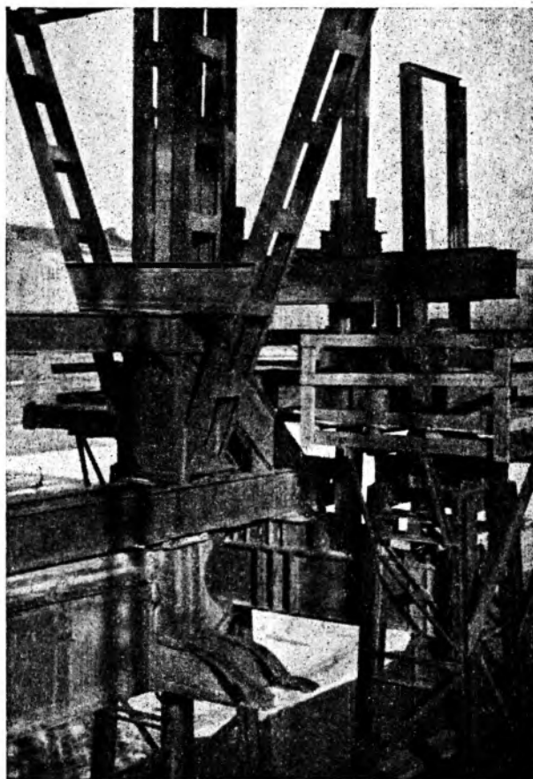
Ryc. 5. Oparcie przęsła środkowego na kozłach po podniesieniu, konstrukcja do podnoszenia.
