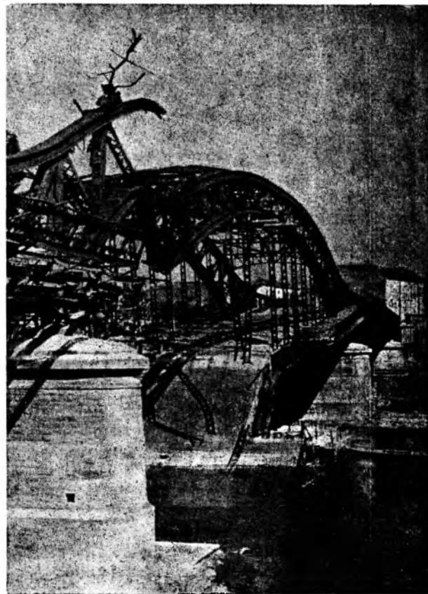
Ryc. 2. Ogólny obraz zniszczeń. Część jezdni jednym końcem wsparta o dno rzeki. Zniszczenie belki łukowej.
