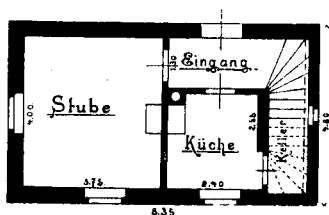
3. Erdgeschoss.
