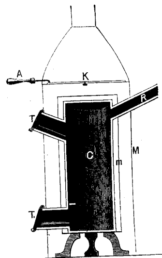
Regulirfüllofen.
