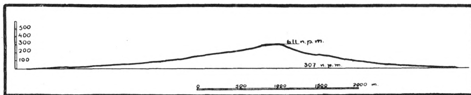
Rys. 1. Przekrój przez Łysicę prostopadły do kierunku wału.
