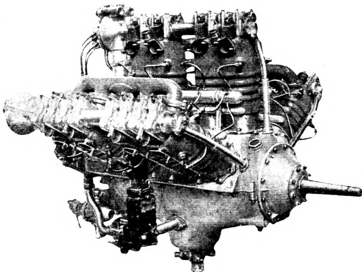
SILNIK SERYJNY „LORRAINE — DIETRICH” 450 MK.
