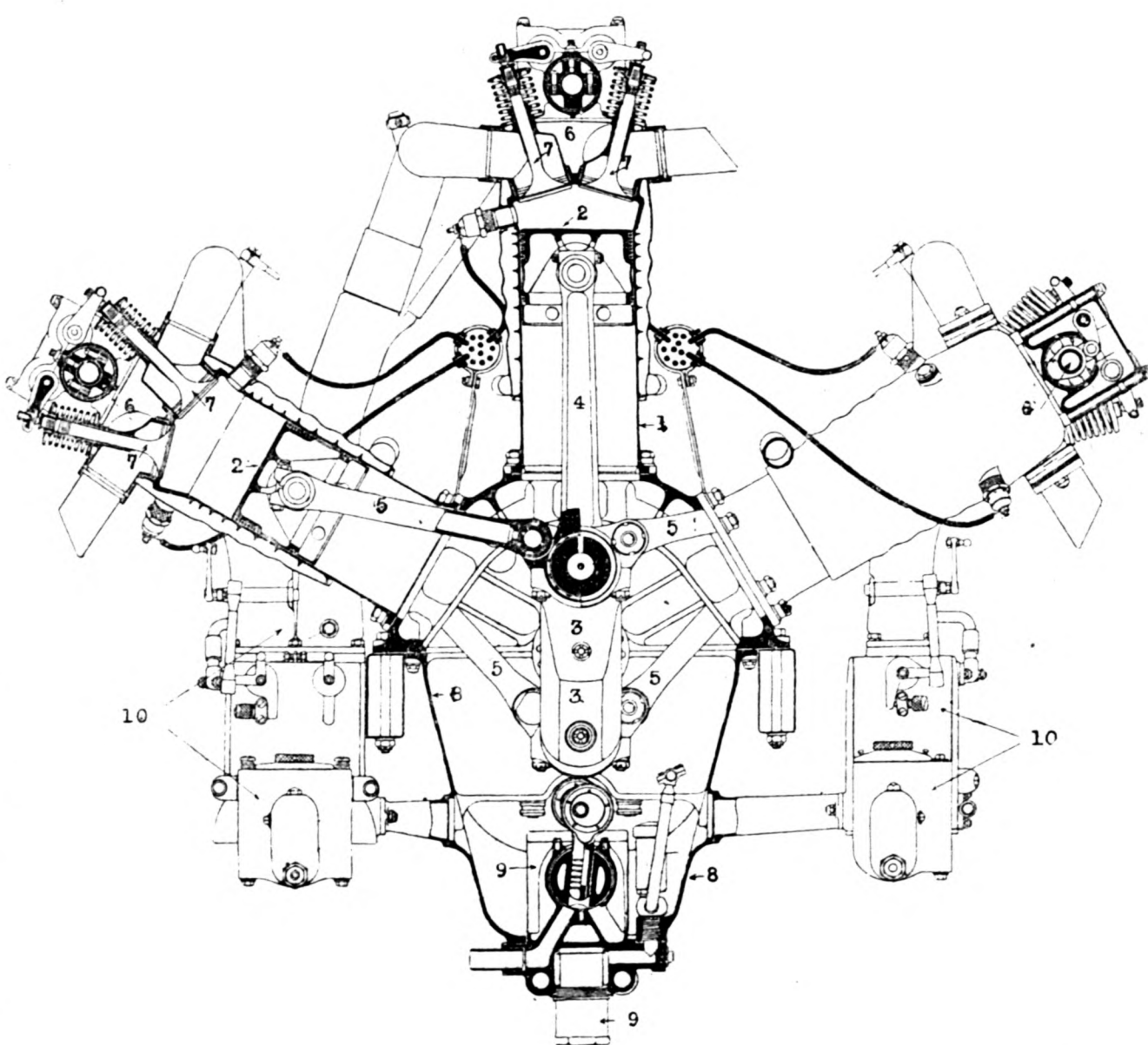
PRZEKRÓJ PIONOWY SILNIKA „LORRAINE—DIETRICH” 450 MK.
