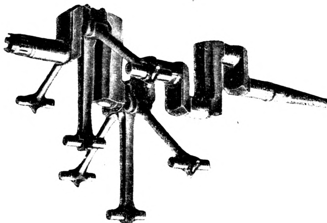
WAŁ KORBOWY SILNIKA „LORRAINE—DIETRICH” 450 MK.
