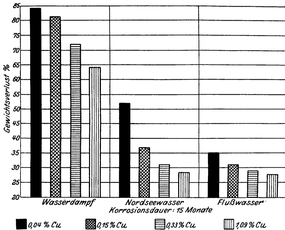
Abb. 5. Korrosionsversuche mit Stählen verschiedenen Kupfergehalts.
