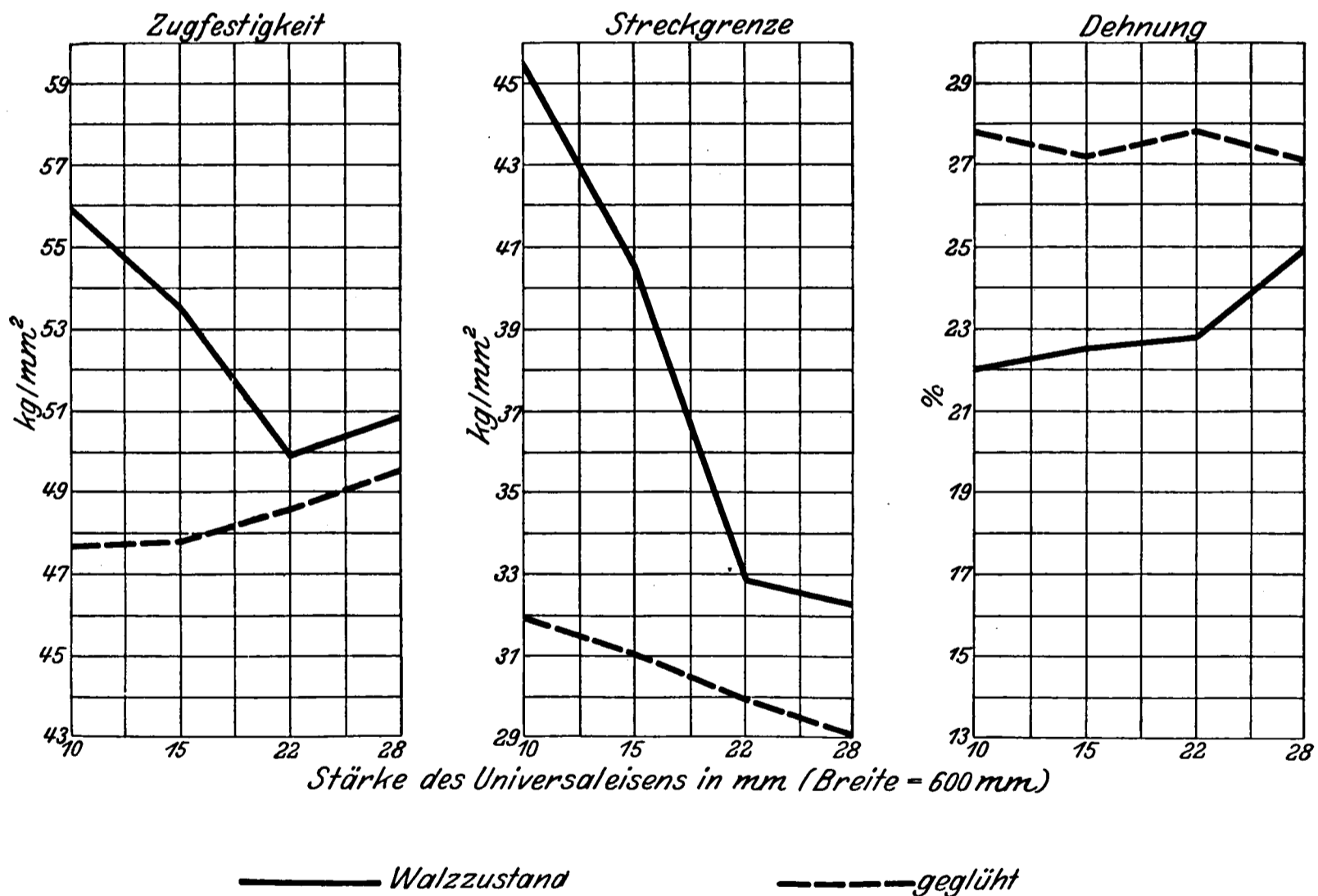
Abb. 2. Abhängigkeit der Festigkeitseigenschaften des Siliziumbaustahls vom Verwalzungsgrad.
