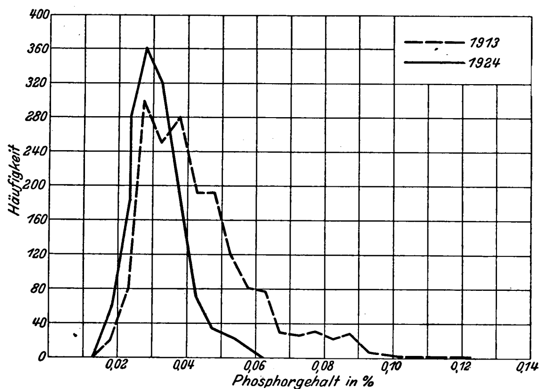
Abb. 18. Häufigkeitskurven des Phosphorgehaltes in der Stahlerzeugung eines Hüttenwerkes 1913 und 1924.
