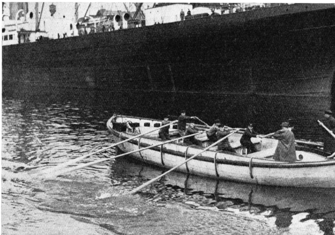
Abb. 10. Das mit einem Eisengewicht entsprechend 145 Personen belastete Boot wird durch 6 Mann gerudert.
