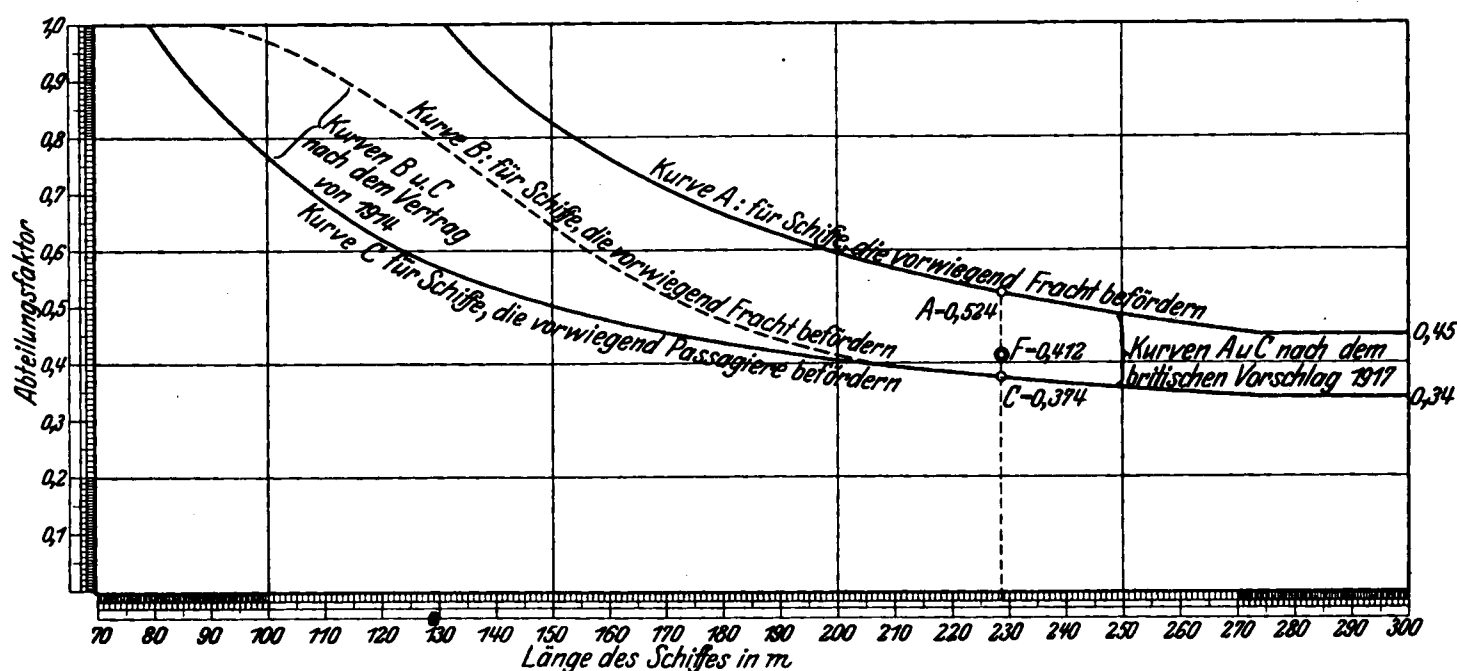
Abb. 3. Kurvenblatt für die Ermittlung des Abteilungsfaktors. Als Beispiel ist die Ermittlung für ein Fracht- und Fahrgastschiff von 228 m eingetragen.
