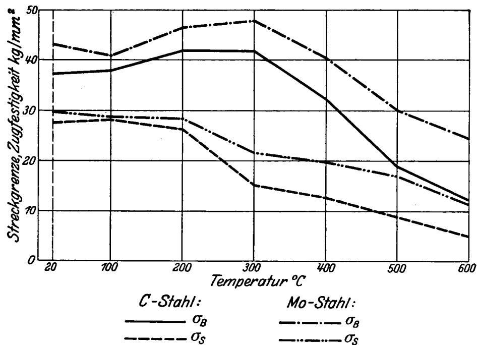
Abb. 9. Einfluß der Temperatur auf Zugfestigkeit und Streckgrenze bei gewöhnlichem und schwach mit Molybdän legiertem Kesselbaustahl (nach N e h l).
