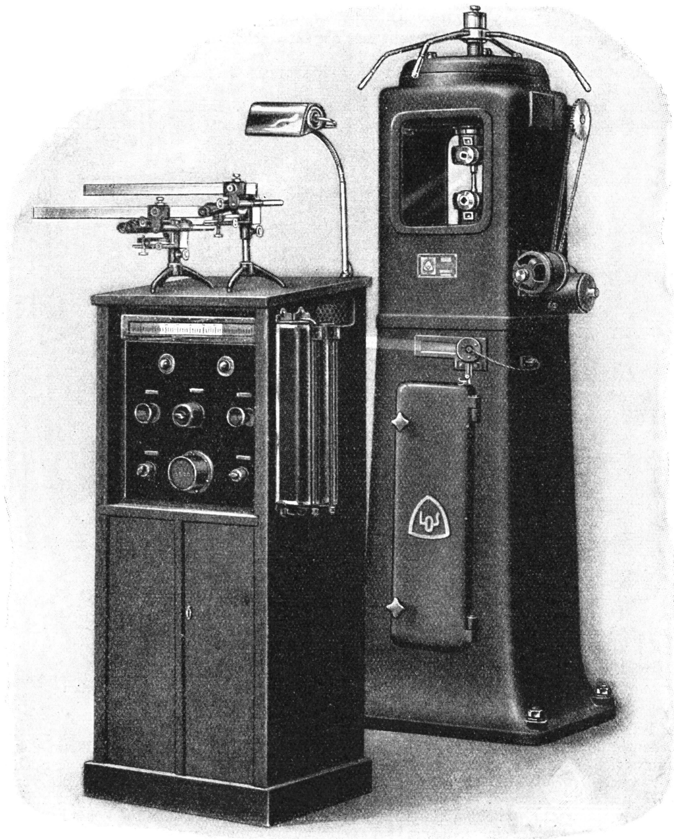
Abb. 1. Dauerprüfmaschine für kombinierte statische und dynamische Belastungen (Torsionswechselbelastung).
