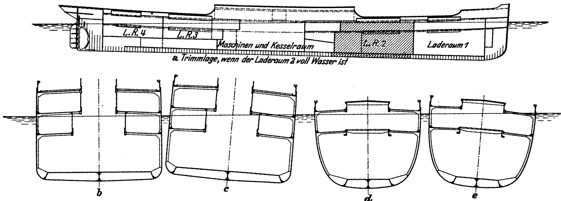
Abb. 1. Frachtfahrgastschiff von 97,50 m Länge.
