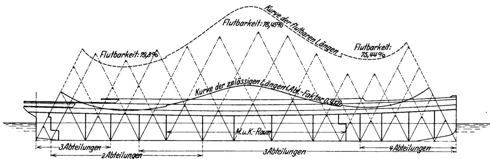
Abb. 5. Dasselbe Schiff wie Abb. 4, aber mit 14 Schotten, wie es gebaut wurde. Bei den angenommenen Flutbarkeiten können fast überall 3 beliebige Abteilungen vollaufen, im Vorschiff sogar 4 Abteilungen.
