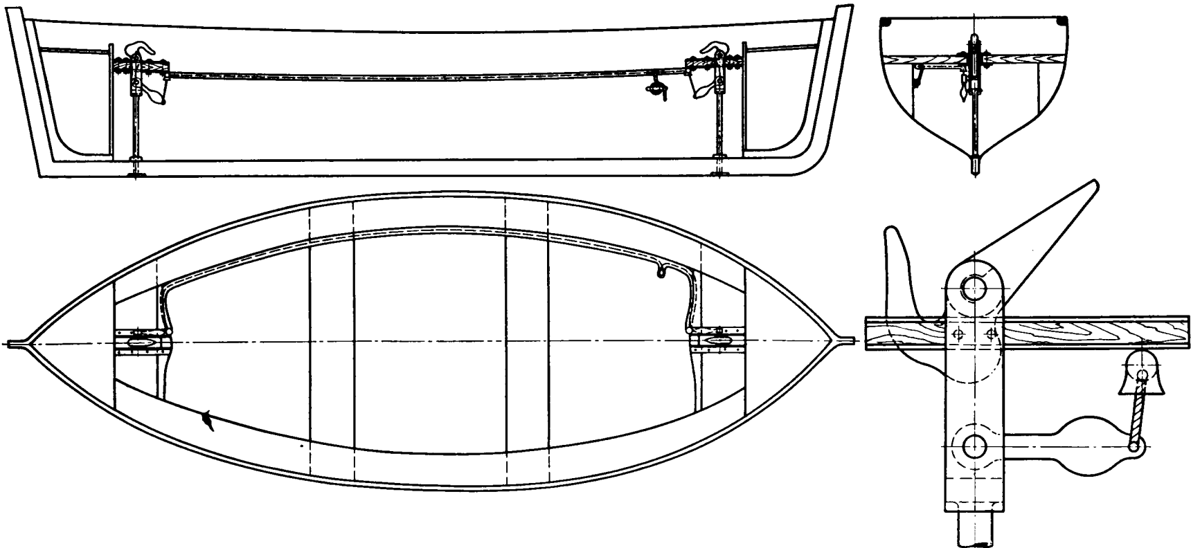
Abb. 2. Normale Anordnung einer Ristauschen Boot-Slipvorrichtung im Rettungsboot.
