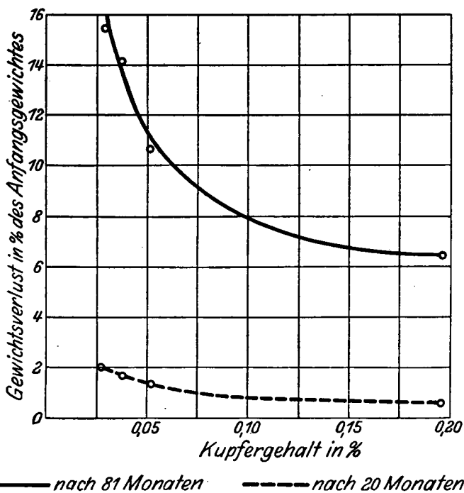
Abb. 4. Ergebnisse der Korrosionsversuche an Schwellen aus gekupferten und gewöhnlichem Stahl.
