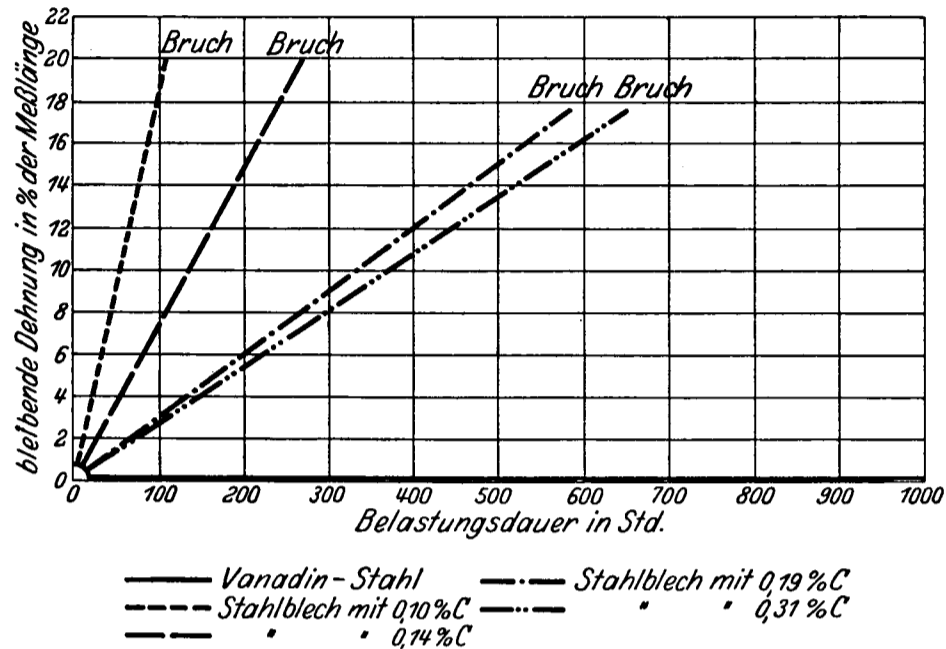
Abb. 11. Dauerstandfestigkeit von Kohlenstoffstählen und Vanadinstahl bei 500° unter 10 kg/mm 2 Belastung.
