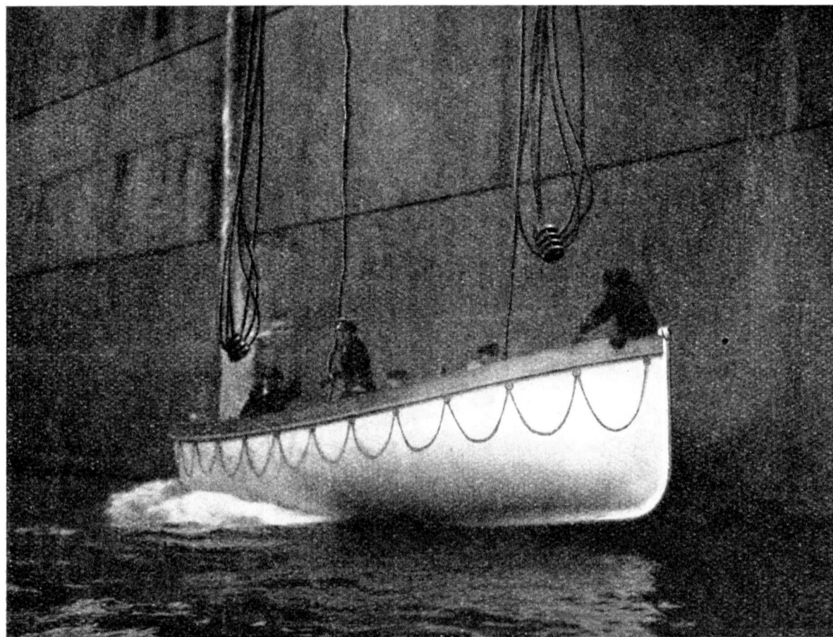
Abb. 3. Fieren des Rettungsbootes bei einer Schräglage von etwa 45^\circ durch die Ristausche Boot-Slipvorrichtung.
