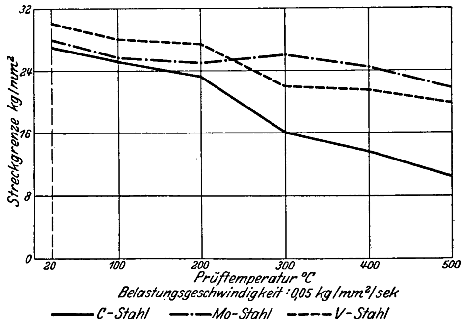
Abb. 10. Einfluß der Temperatur auf die Streckgrenze bei Vanadin- und Molybdän-Kesselbaustählen (nach Prömper und Pohl).
