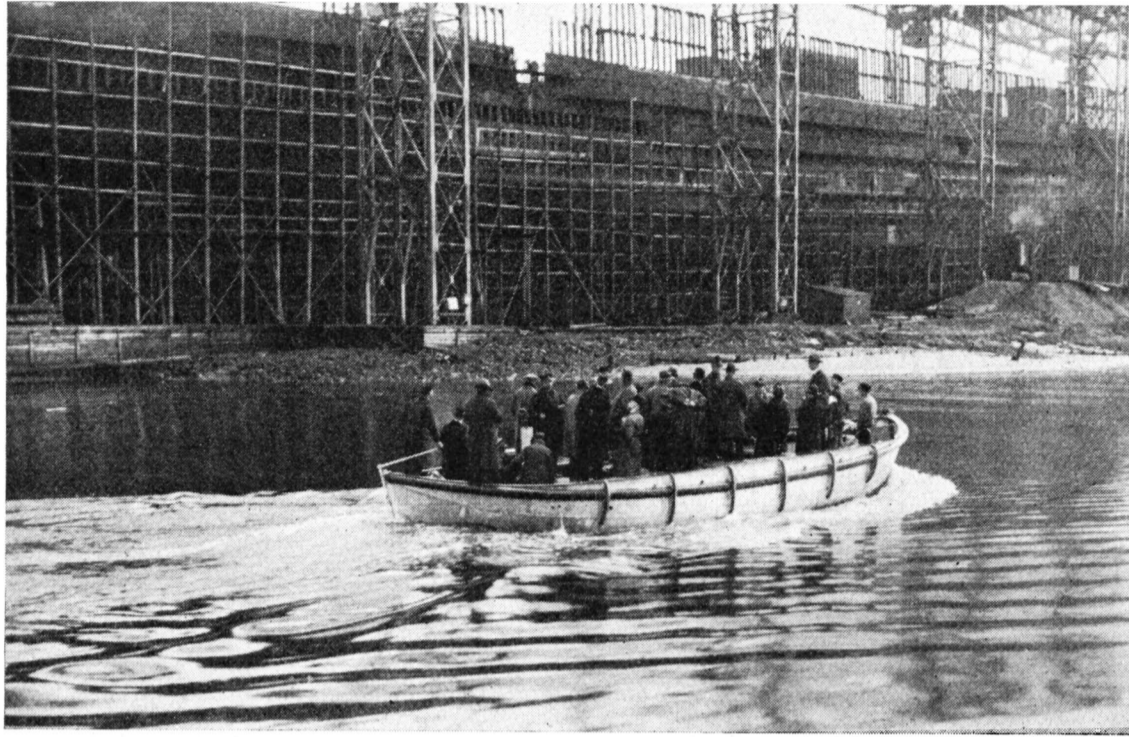
Abb. 9. Das mit Eisen entsprechend dem Gewicht von 145 Personen belastete und außerdem mit ca. 30 Zuschauern besetzte Boot macht eine Probefahrt mit 6 Knoten Geschwindigkeit.
