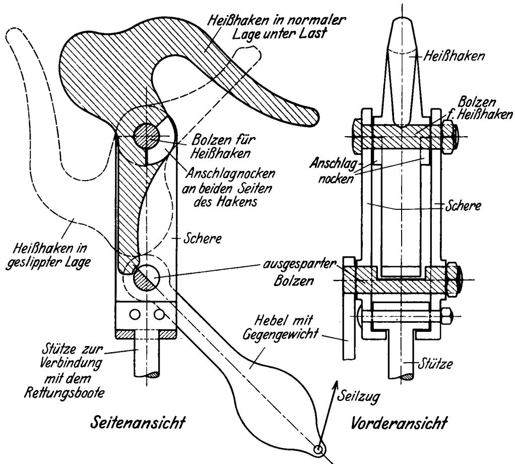
Abb. 1. Boot-Sliphaken nach Patent „Ristau“.
