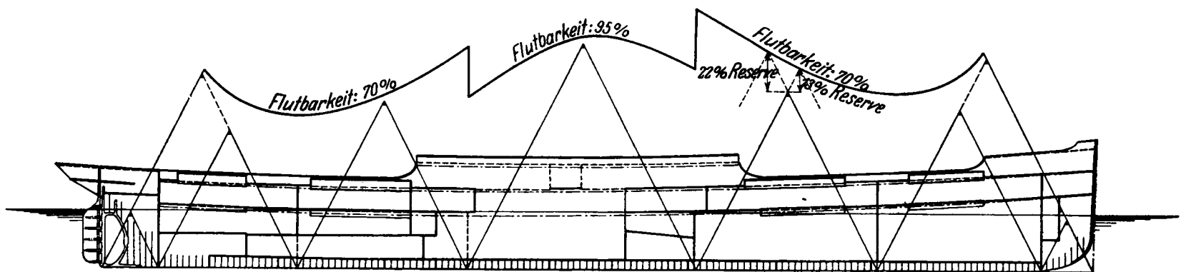
Abb. 2. Frachtfahrgastschiff von 97,50 m Länge. Kurve der flutbaren Längen und Schotteinteilung. Die Flutbarkeiten sind den Vorschriften der Seeberufsgenossenschaft 1908 entnommen. Die beiden vorderen, die beiden hinteren oder eine beliebige Abteilung kann leck werden.
