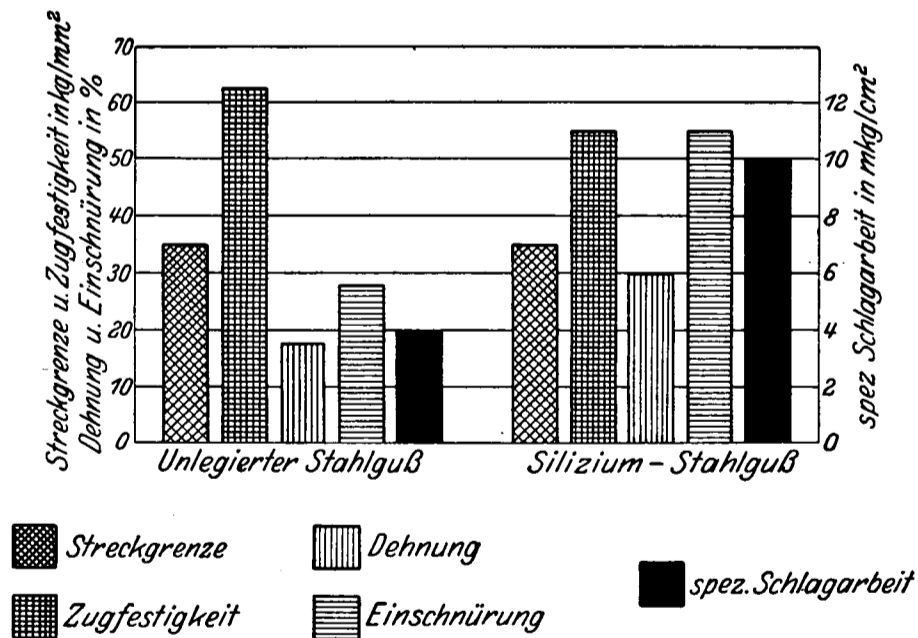
Abb. 12. Festigkeitseigenschaften von Siliziumstahlguß.
