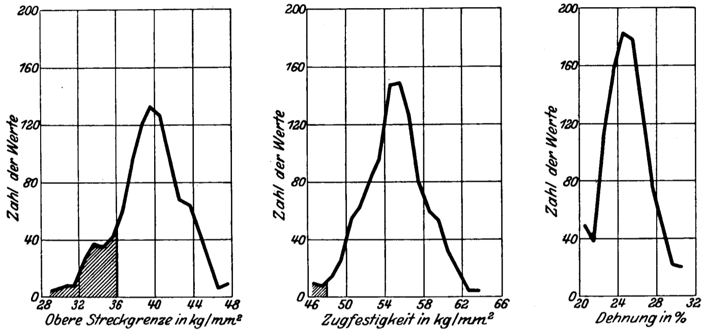
Abb. 1. Häufigkeitskurve der Festigkeitswerte von Siliziumbaustahl.
