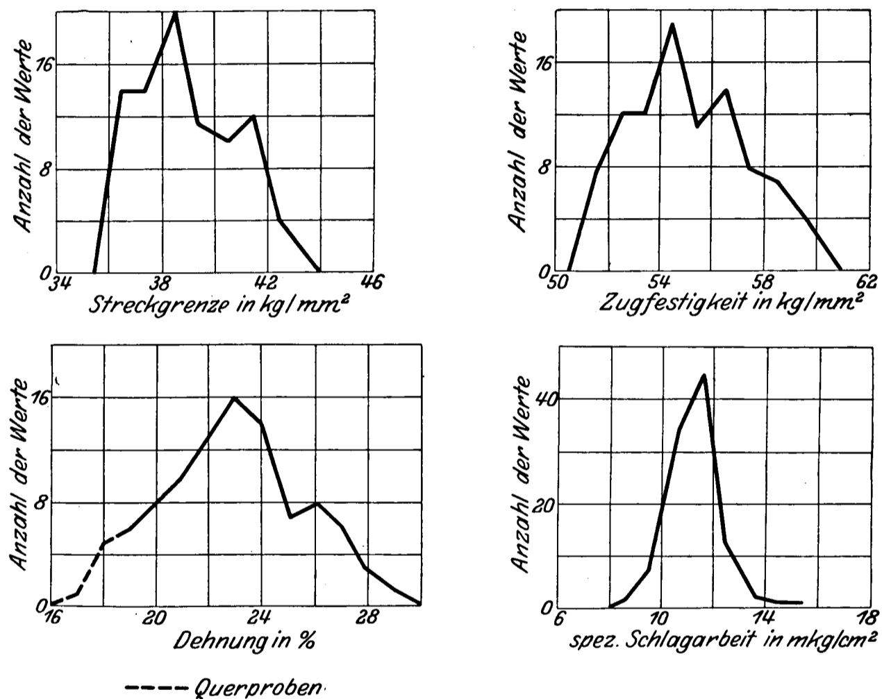
Abb. 3. Häufigkeitskurven der Festigkeitswerte von Union-Baustahl.
