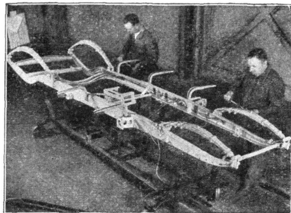
2. Umocowanie resorów.
