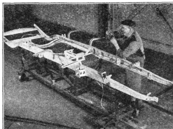
1. Montaż przewodów smarowniczych i hamulcowych.
