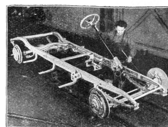
5. Wstawianie kierownicy.
