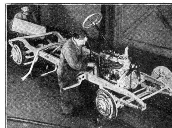
8. Montaż przewodów wydechowych i zbiornika paliwa.
