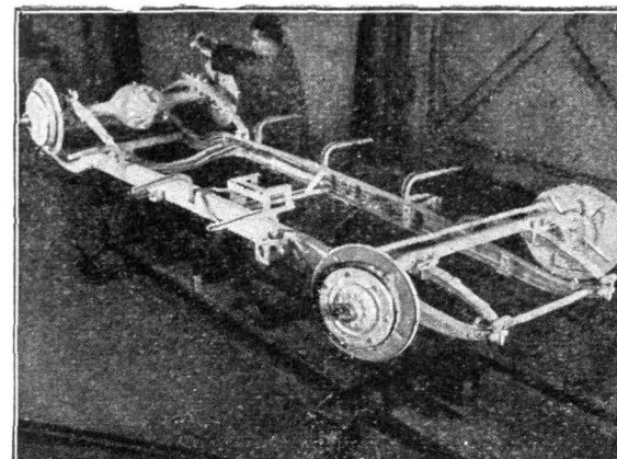
4. Umocowanie tylnego mostu.
