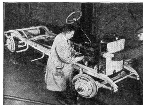
9. Montaż chłodnicy.
