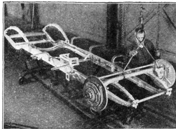
3. Wstawianie przedniej osi.
