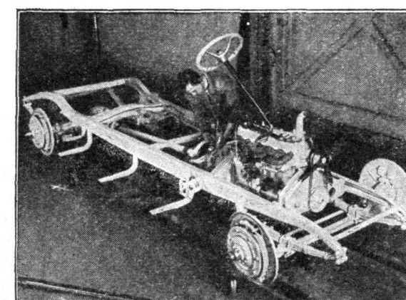
7. Wstawianie wału kardanowego.
