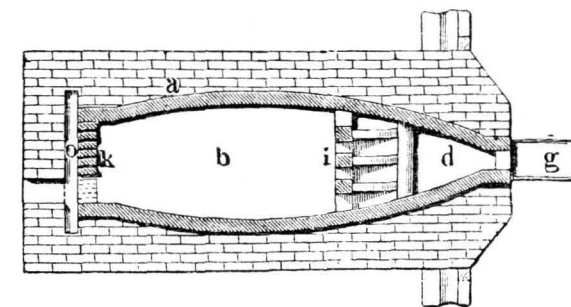
6. Jednokomorowy piec płomienny (przekrój podł. i poprz.).
