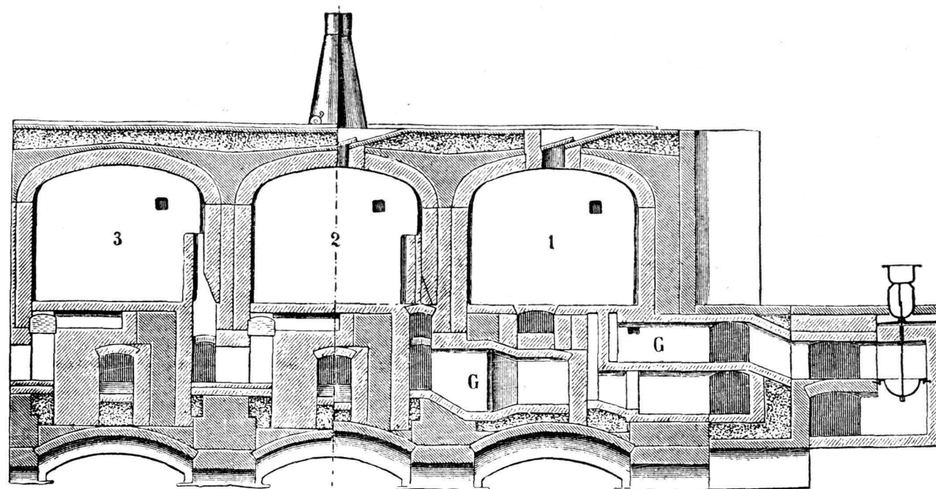
2. Piec kanałowy Mendheima.
