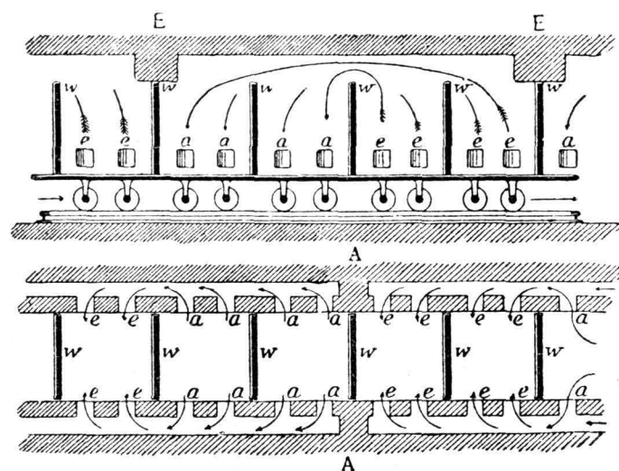
3. i 4. Piec tunelowy Faugeron (schemat i widok ogólny).
