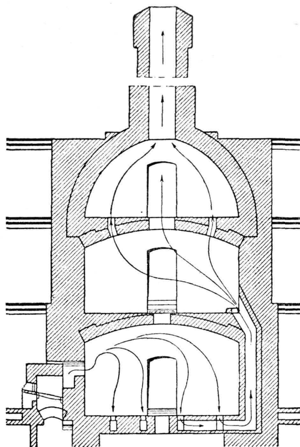
1. Piec płomienny piętrowy.
